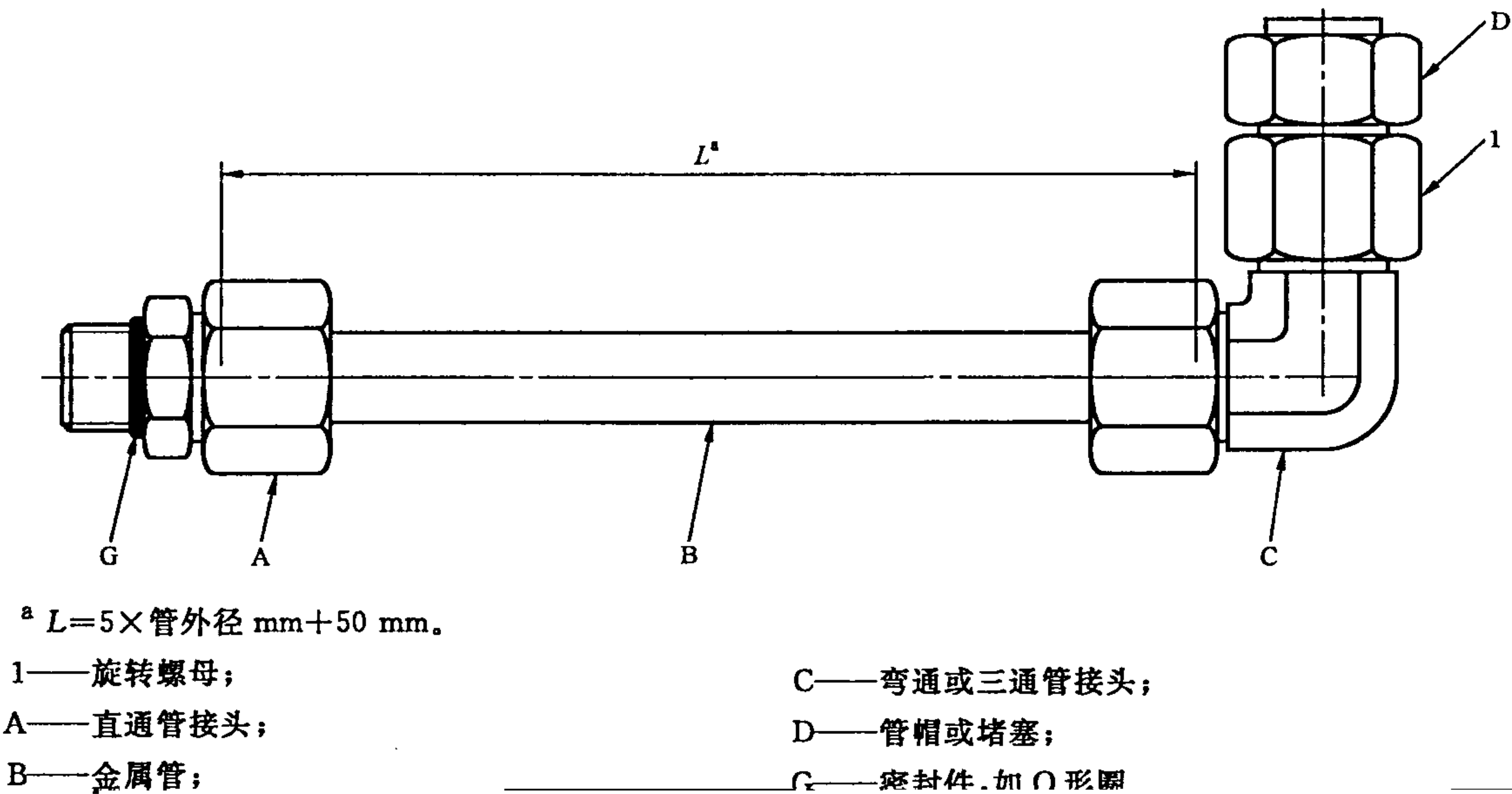
图 B.1 管连接试验总成——1 型
